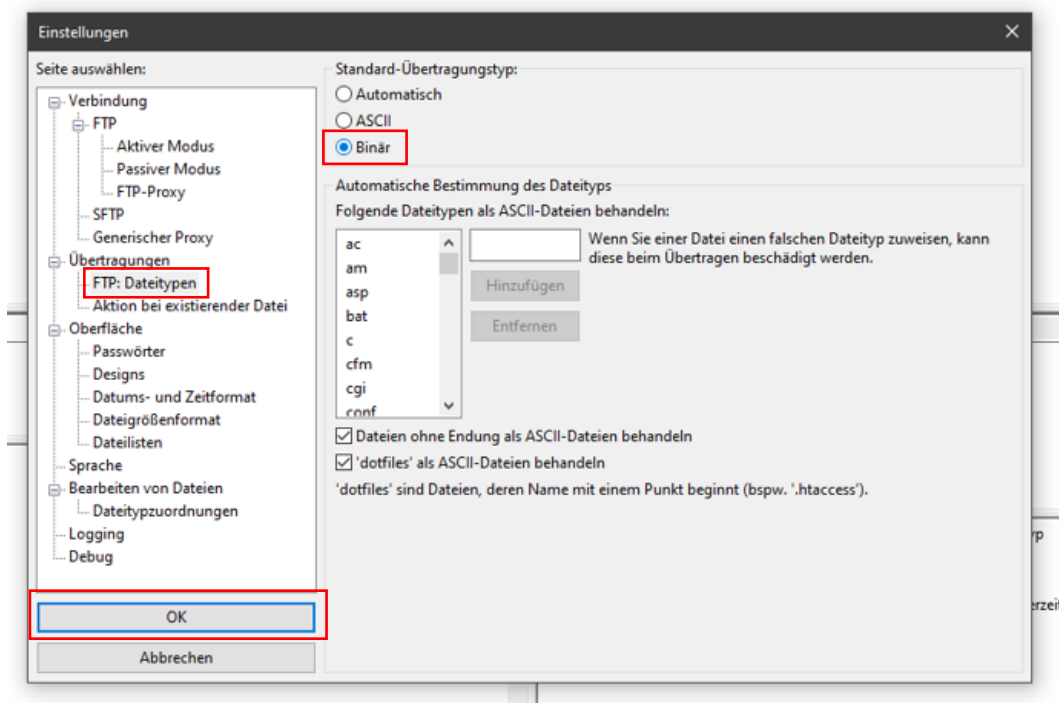
Abbildung 27: Binärer Datentransfer
