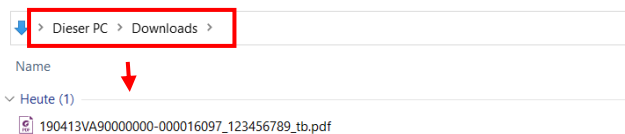
Abbildung 21: Heruntergeladene PDF-Datei
